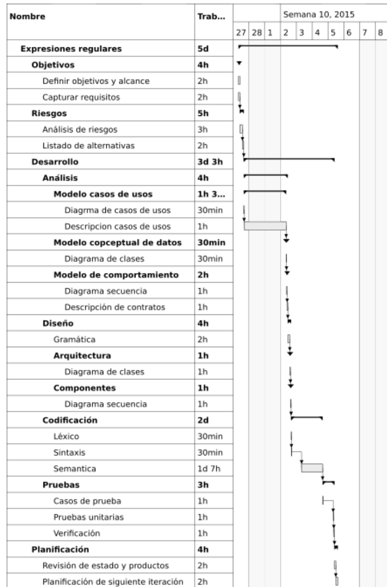
Figura 2.14: Expresiones regulares: 27/02/2015 - 05/03/2015
