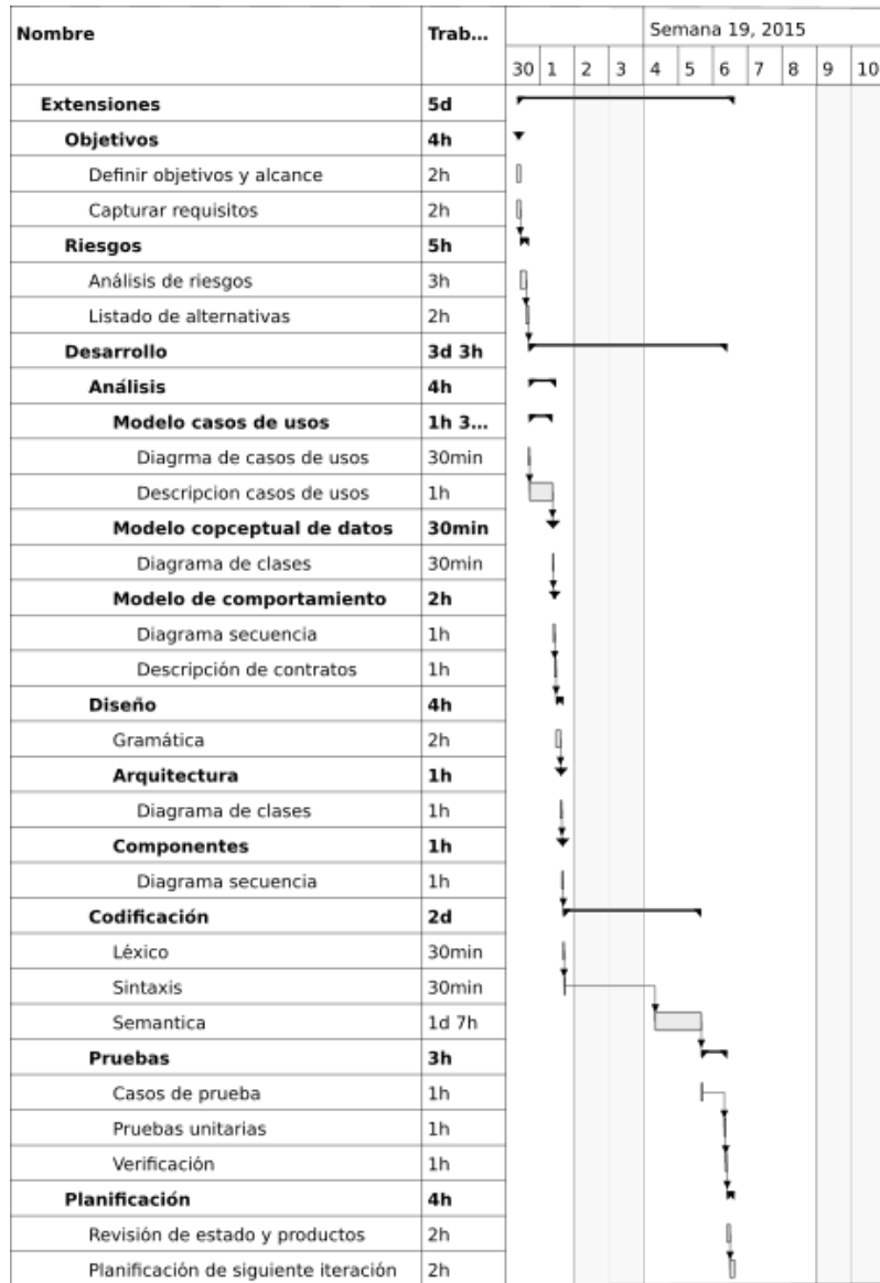
Figura 2.25: Extensiones: 30/04/2015 - 06/05/2015
