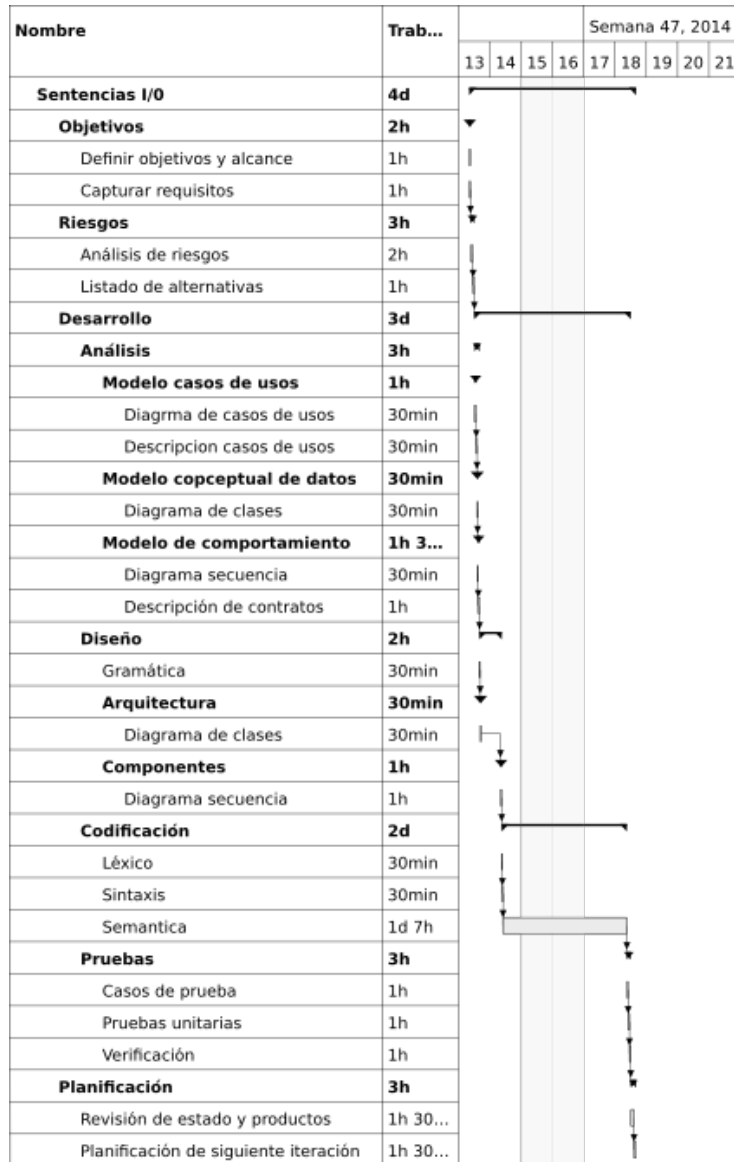
Figura 2.3: Sentencias I/O: 13/11/2014 - 18/11/2014
