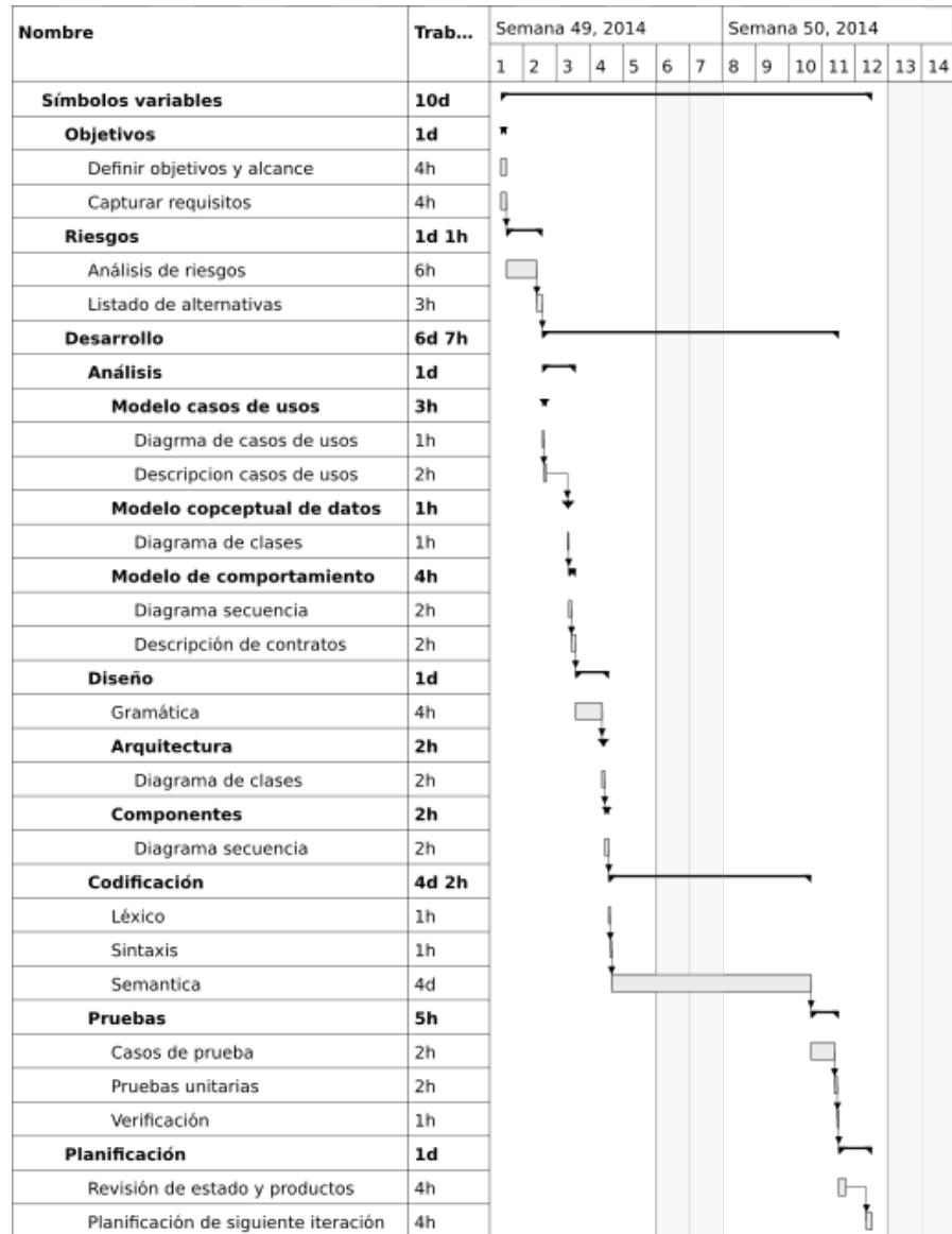
Figura 2.6: Símbolos variables: 01/12/2014 - 14/12/2014
