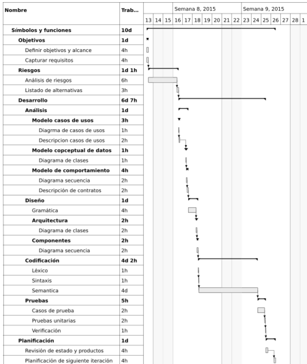
Figura 2.13: Símbolos funciones: 13/02/2015 - 26/02/2015
