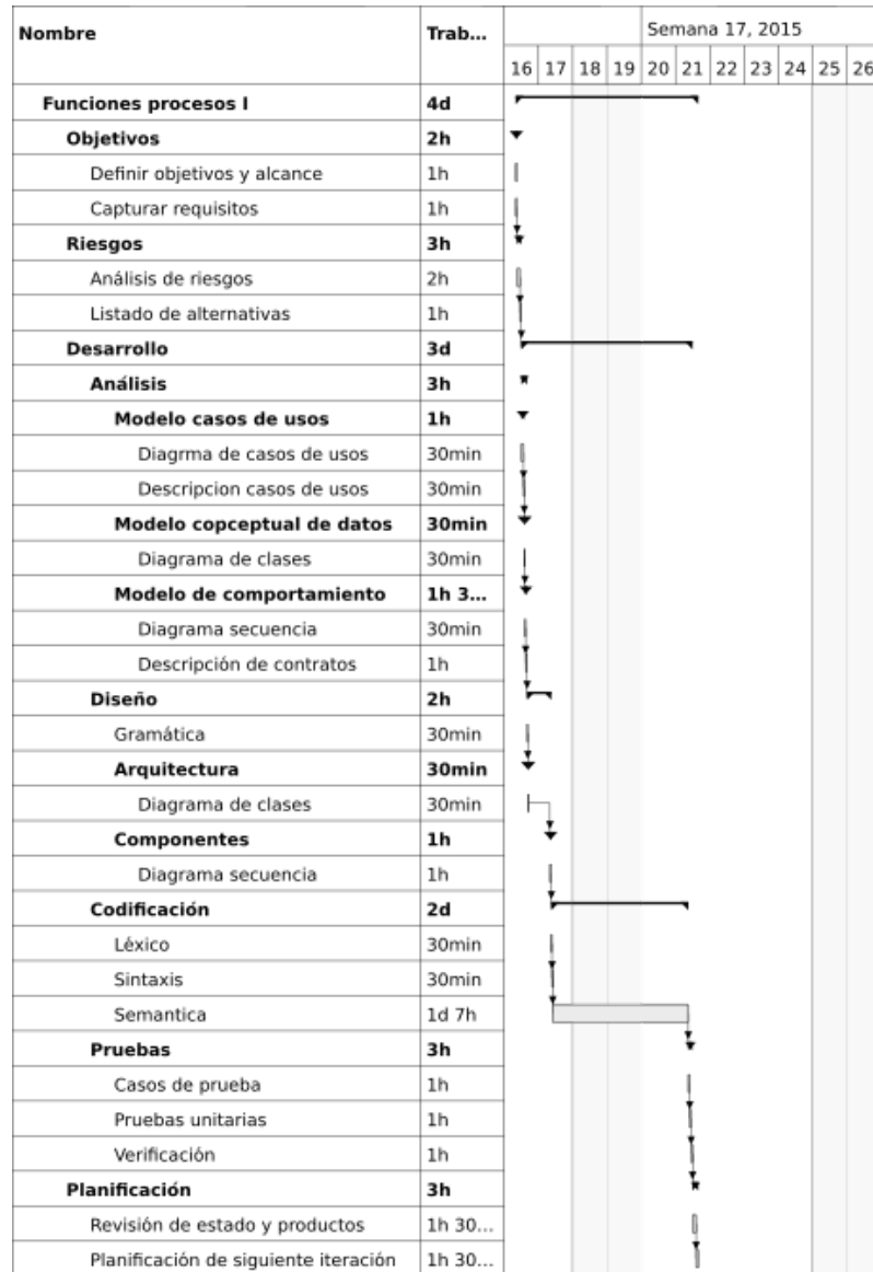
Figura 2.22: Procesos I: 16/04/2015 - 21/04/2015
