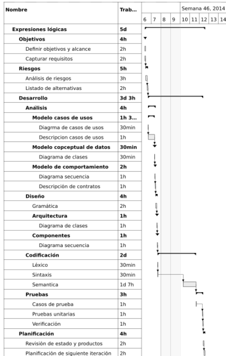
Figura 2.2: Exp. lógicas: 06/11/2014 - 12/11/2014
