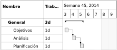
Figura 2.1: General: 03/11/2014 - 05/11/2014
