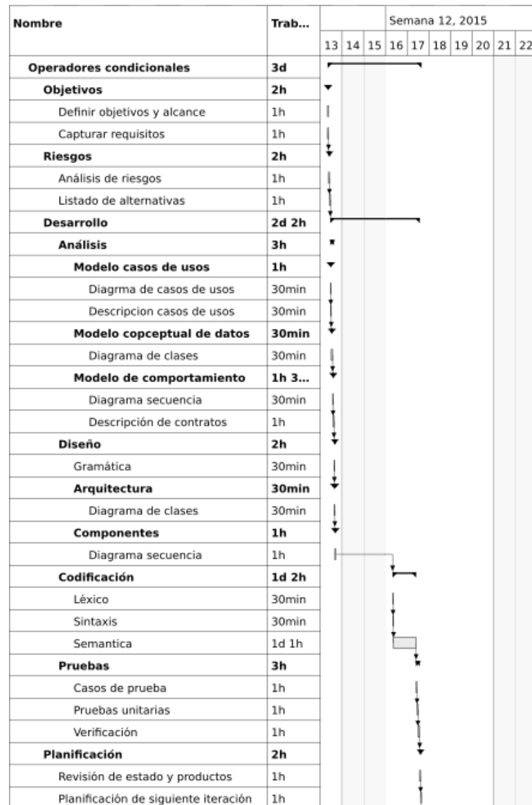
Figura 2.16: Expresiones condicionales: 13/03/2015 - 17/03/2015
