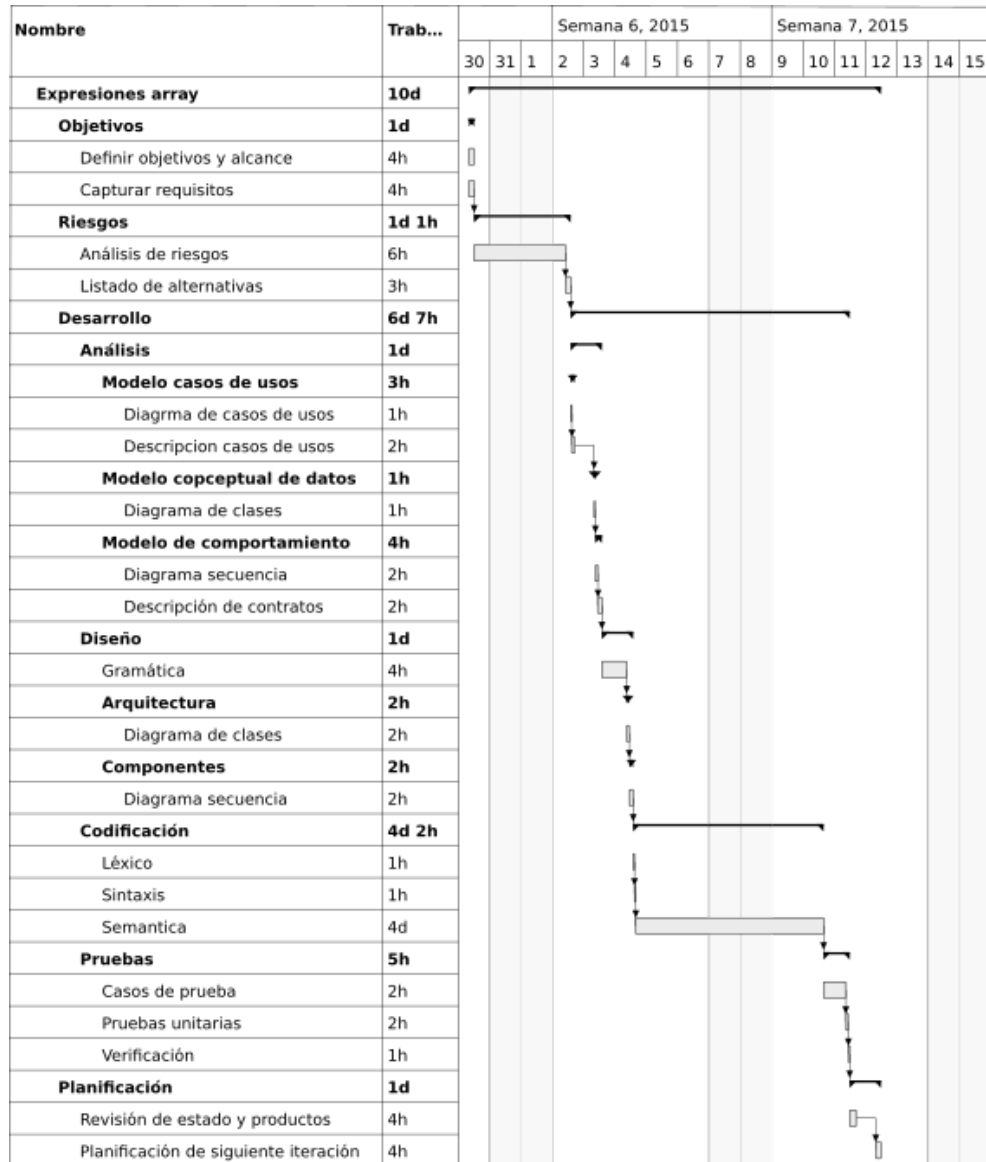
Figura 2.12: Expresiones array: 30/01/2015 - 12/02/2015
